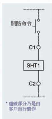
接線圖
